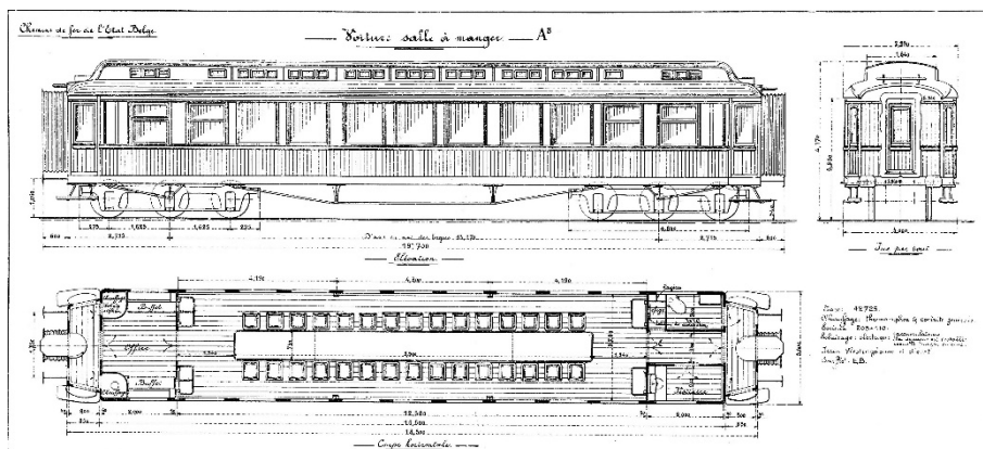
Schéma de la voiture salle à manger A2 (Réf. C3456 p.266)
